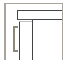
FRONTALE ANTA CON MANIGLIA FRONTALE FRONTAL / DOOR WITH FRONT HANDLE
